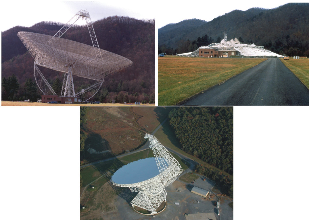
Obrázek 11.4: Nahoře: Původní velký radioteleskop v NRAO, Green Bank, 15. listopadu 1988 a vpravo následující den, po zhroutilí. Dole: Zničený radioteleskop nahradil nový přístroj – Robert C. Byrd Green Bank Telescope. Foto: Richard Porcas, NRAO.
