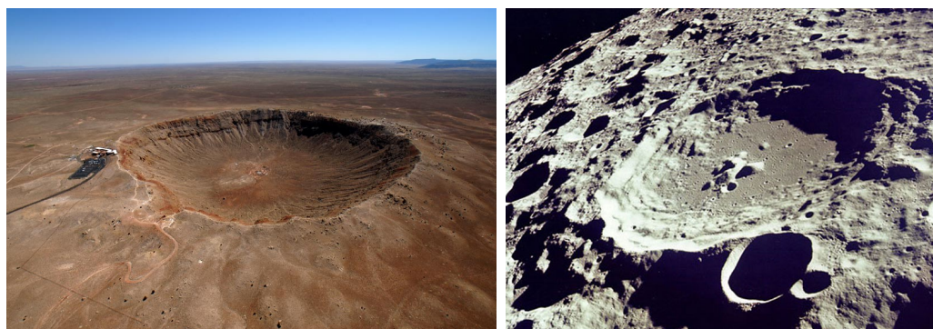
Obrázek 12.3: Impaktní krátery. Vlevo: Barringerův kráter v Arizoně, USA. Vpravo: Měsíční kráter Daedalus. Zdroj: National Geographic, NASA.
