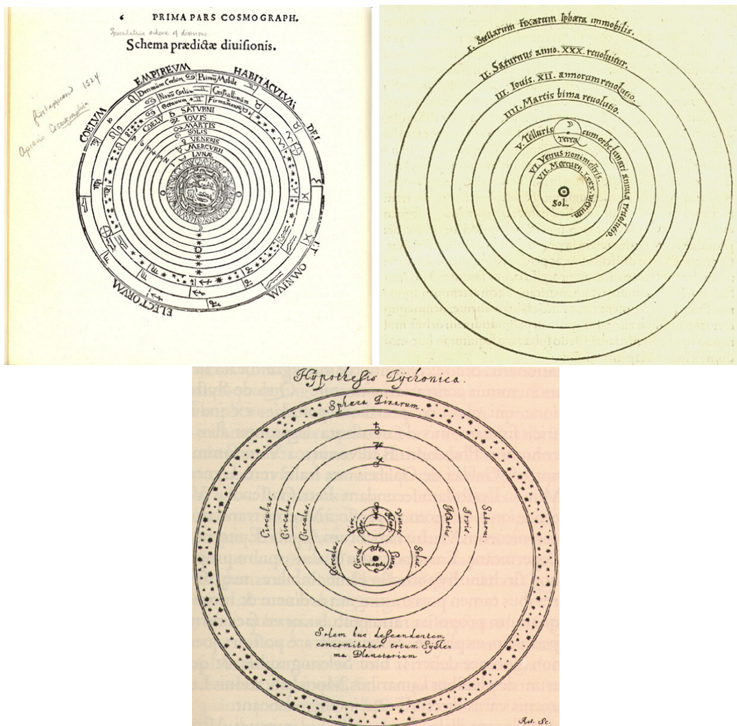
Obrázek 12.36: Modely Sluneční soustavy. Vlevo nahoře geocentrická soustava (Christian Aristotelian Cosmos. Peter Apian: Cosmographia) , vpravo nahoře heliocentrická (M. Koperník: De revolutionibus orbium coelestium) a dole smíšený systém, který navrhl Tycho Brahe. Zdroj: wikipedia.
