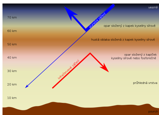
Obrázek 12.10: Skleníkový jev – příčina extrémních podmínek na Venuši. Zdroj: wikipedia.
