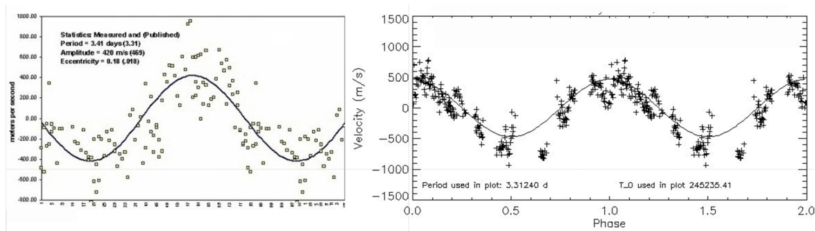
Obrázek 13.9: Křivka radiálních rychlostí hvězdy \tau Boo jasně ukazuje přítomnost exoplanety. Měření byla provedena skupinou amatérských astronomů v letech 2000 (obrázek vlevo) a 2004. Převzato z http://www.spectrashift.com .
