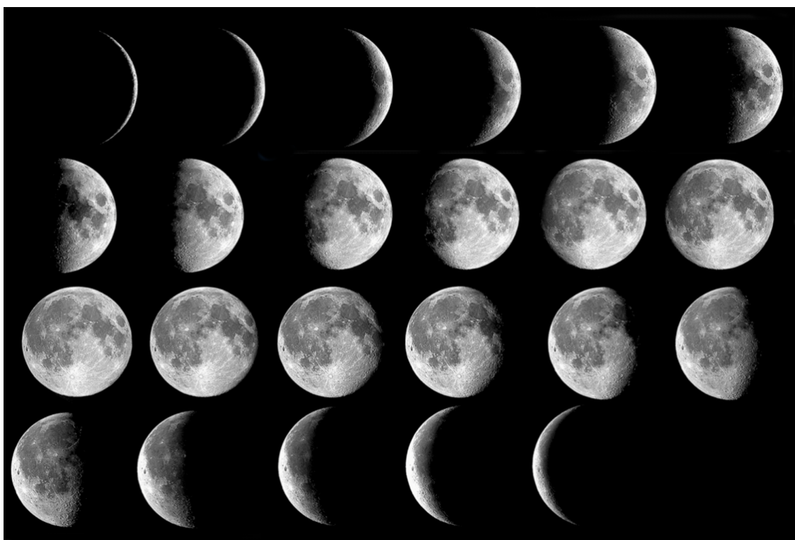
Obrázek 6.9: Fáze Měsíce. Foto: A. Cidado.
