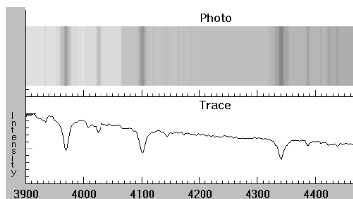
Obrázek 8.7: Horní část obrázku ukazuje fotografii hvězdného spektra v rozsahu 390 až 450 nm. Pro zpracování spektra je nutné proměřit zaznamenanou intenzitu v závislosti na vlnové délce. Dříve se takové měření provádělo ručně. Dnes je to záležitost softwaru, který projde digitální fotografií spektra od jednoho okraje k druhému a zaznamenané intenzity vynese do grafu v dolní části obrázku. Převzato z Projektu CLEA, http://www3.gettysburg.edu/marschal/clea/cleahome.html .
