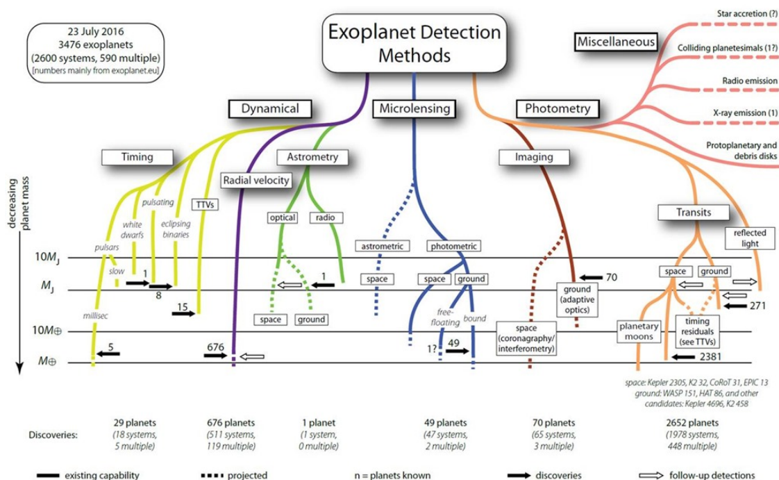
Obrázek 13.3: Diagram metod detekce exoplanet. Stav k 23. 7. 2016. Převzato z http://exoplanetes.esep.pro .
