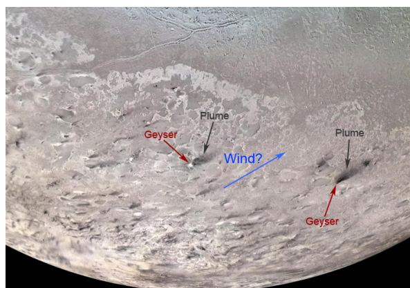
Obrázek 12.31: Gezíry tekutého dusíku poblíž jižního pólu Tritonu. Jak se vyvržený materiál snáší zpět na povrch, naznačuje převažující směr proudění atmosféry. Zdroj: NASA.
