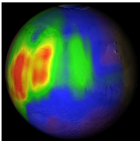
Obrázek 14.7: Oblasti s největším zaznamenaným výskytem metanu na povrchu Marsu. Zdroj: tisková zpráva NASA 09-006.
