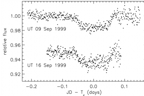
Obrázek 13.10: První zaznamenané tranzity exoplanety HD 209458 b. Zdroj: Charbonneau et al. (2000).
