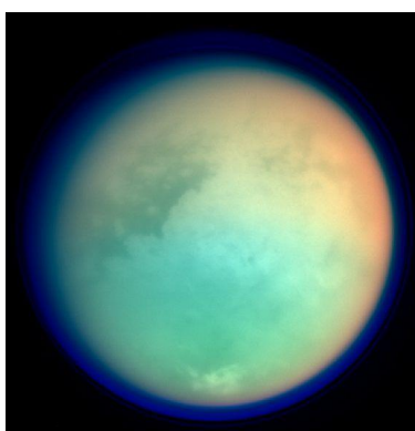
Obrázek 12.28: Složený snímek Titanu (v IR a UV) ze sondy Cassini 26. října 2004. Zdroj: NASA.
