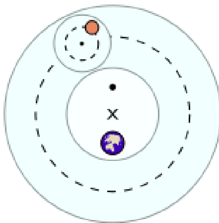
Obrázek 12.35: Ptolemaiův model Sluneční soustavy. Planeta obíhá kolem Země na epicyklu (malá čárkovaná kružnice) a deferentu (velká čárkovaná kružnice). Země je umístěná excentricky a na protější straně vůči uvažovanému středu soustavy (x) je ekvant (černý bod). Planeta, respektive střed epicyklu, pak obíhá vůči ekvantu s konstantní rychlostí. Zdroj: wikipedia.
