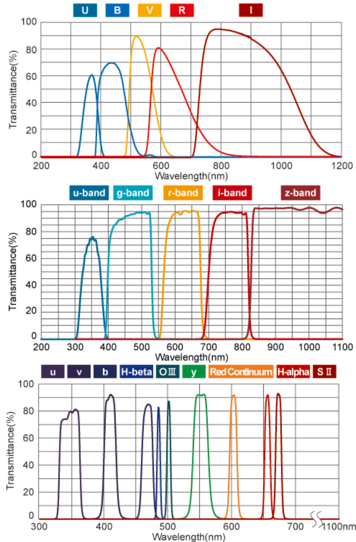
Obrázek 9.4: Ukázka křivek propustnosti filtrů různých fotometrických systémů. Nahoře je nejběžnější, širokopásmový Johnsonův systém UBVRI . Uprostřed systém používaný pro přehlídkový projekt SDSS a dole několik úzkopásmových filtrů. Zdroj: http://www.asahi-spectra.com .
